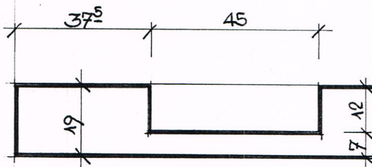
ANSICHT LINTEN
