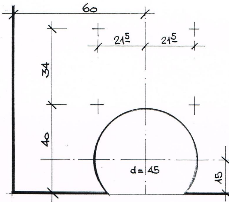
ANSICHT FRONT
